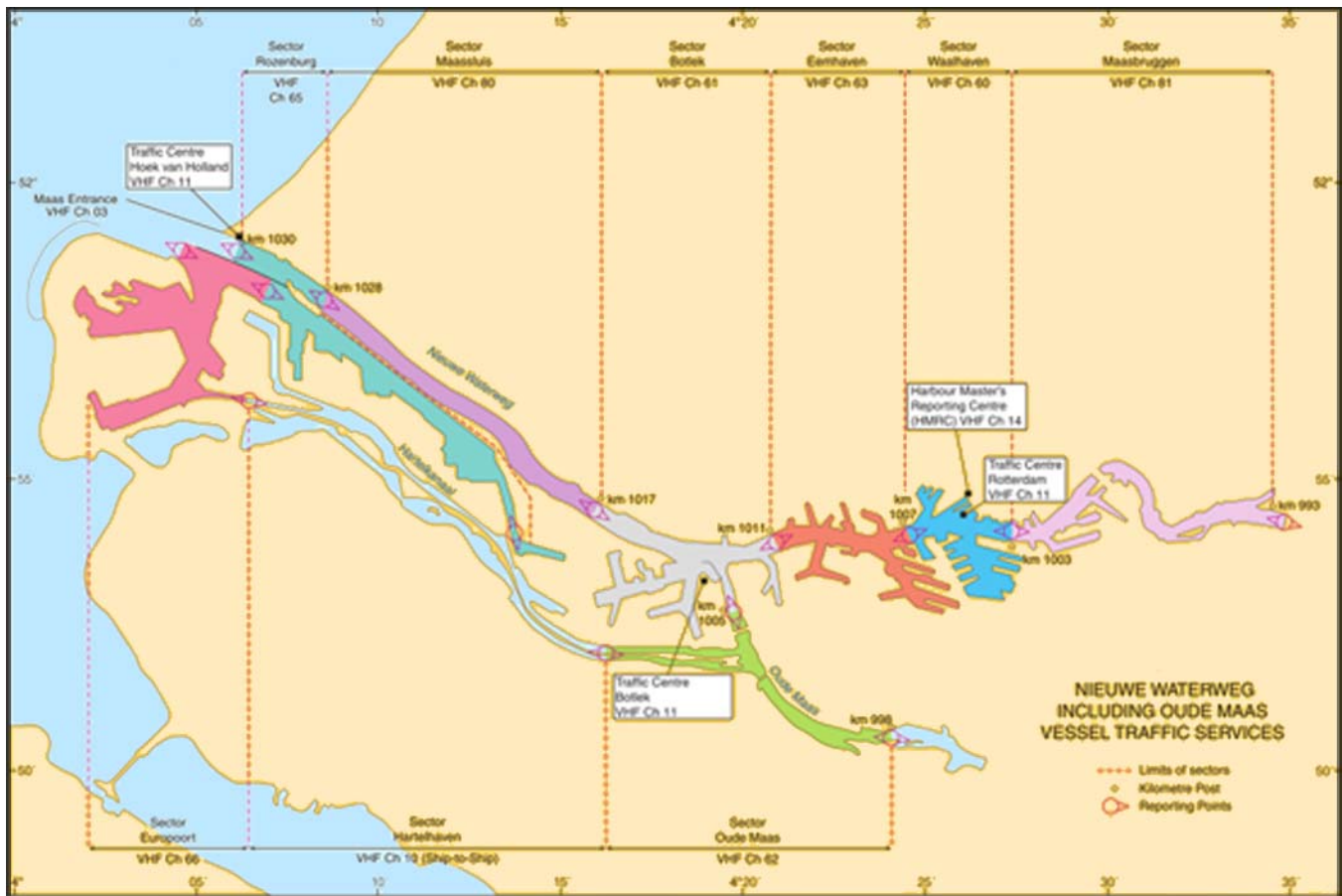
VTS for Nieuwe Waterweg to Rotterdam
