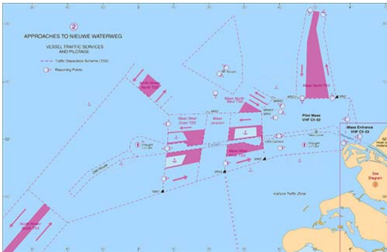
Nieuwe Waterweg TSS
